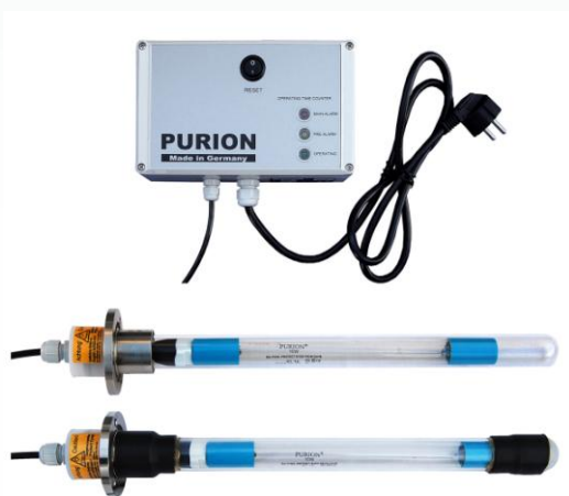
Bild: PURION UV-Set 10 W & optional mit Splitterschutz
